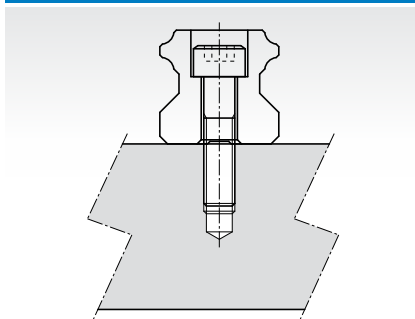
沉头孔型(R型)
