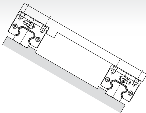
倾斜方式(代码：T)
